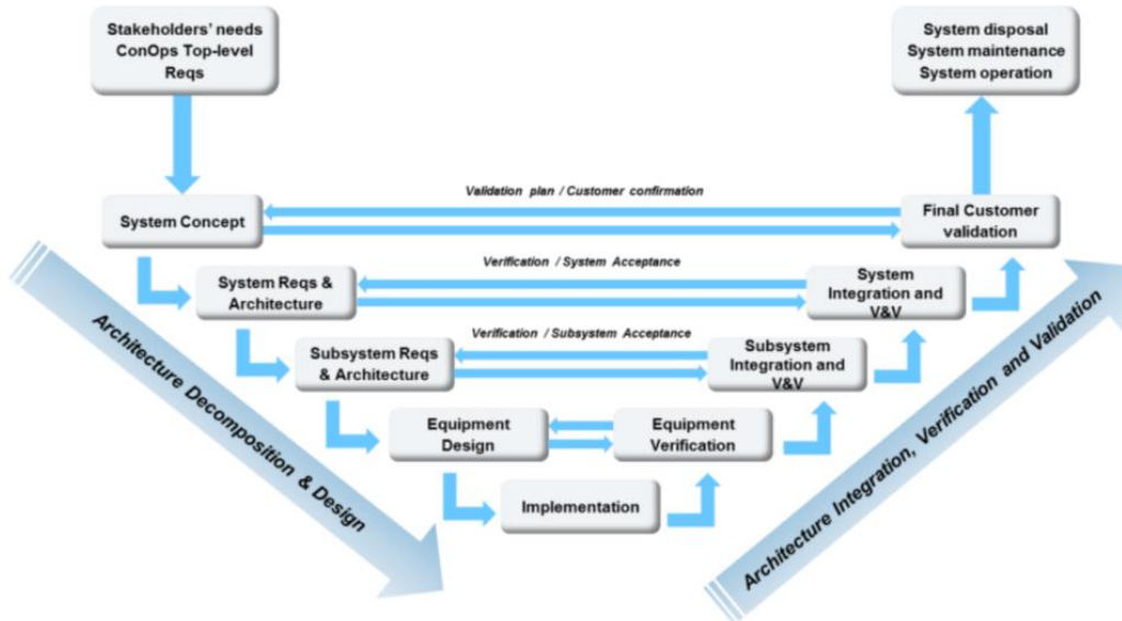
Fig. 1. V-model.
